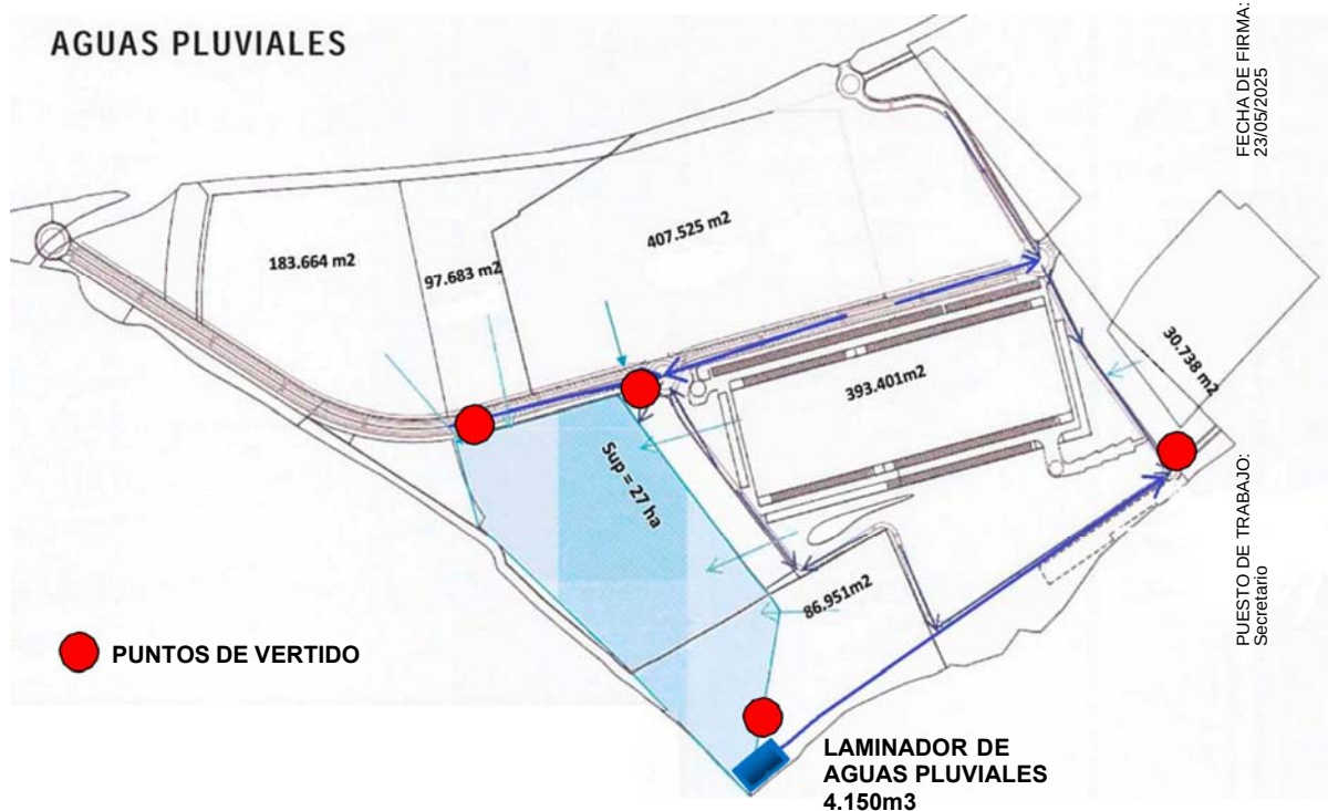
Esquema de red de saneamiento de aguas pluviales proyectada.
